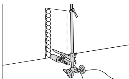
Bodové vrtanie.
